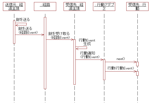
図 4: 経路 Event が引き起こす行動
