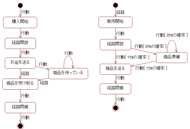
図 6: 購入・販売ステートチャート
